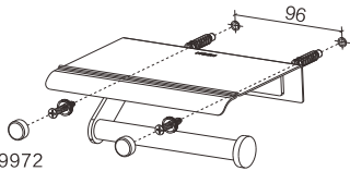
ACC9972 带平台单厕纸架
