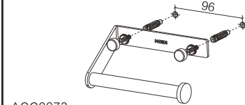
ACC9973 带平台单厕纸架延伸杆
