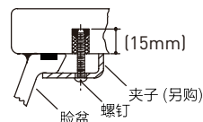
夹子方式
