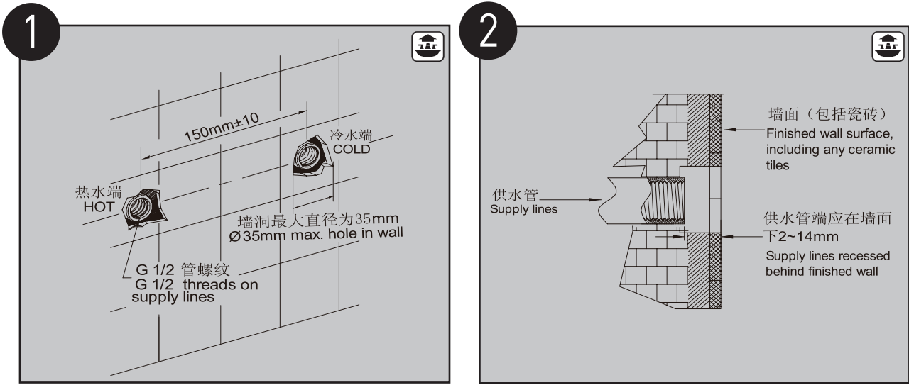
供水管路布置。 Configure supply lines.
