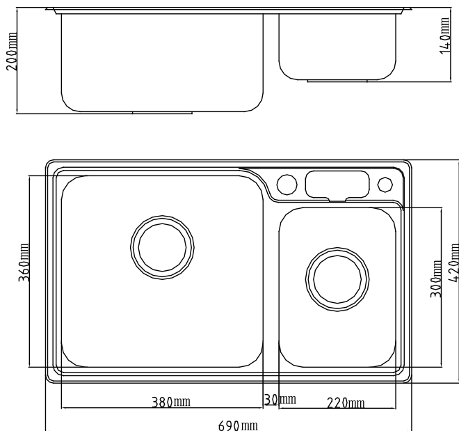
尺寸图
