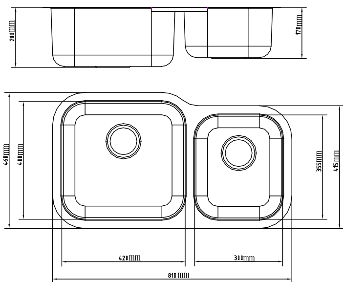
尺寸图
