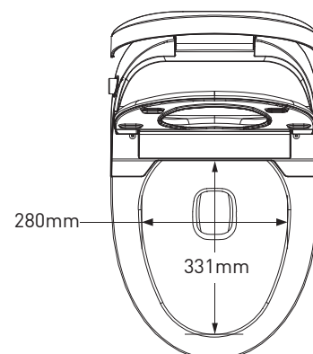
俯视图 Top View
