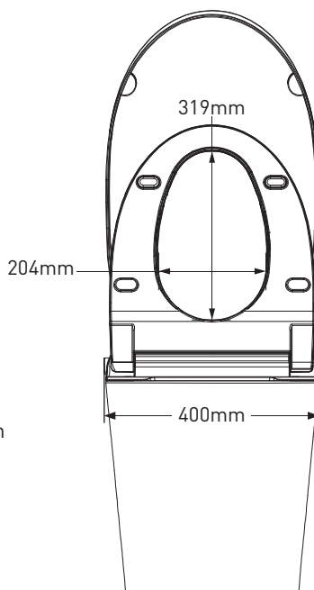
正视图 Front View
